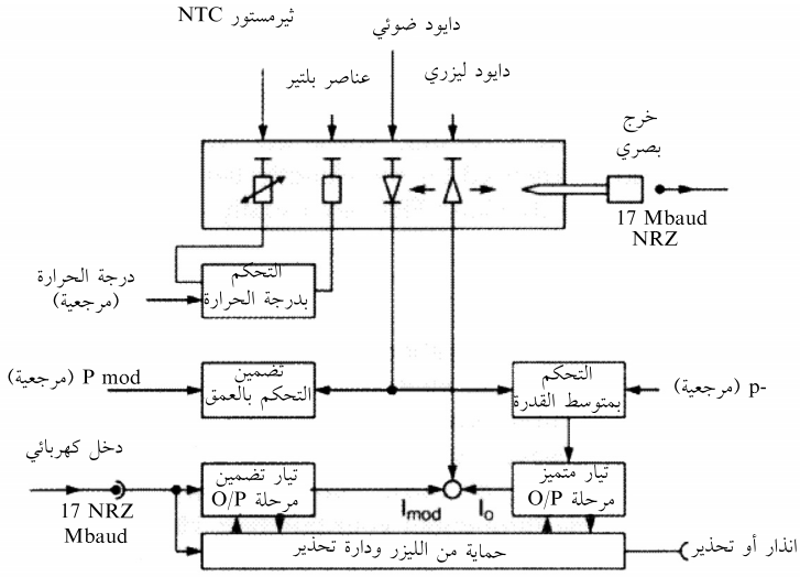
الشكل 9-9 رسم تخطيطي لفعلية جهاز إرسال بصري.
